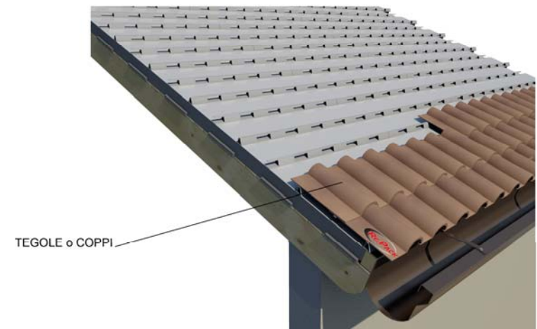
8) ANCORAGGIO TEGOLE o COPPI
