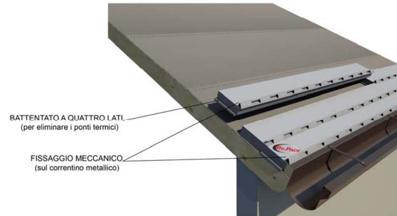
6) FISSAGGIO REFLECTO
