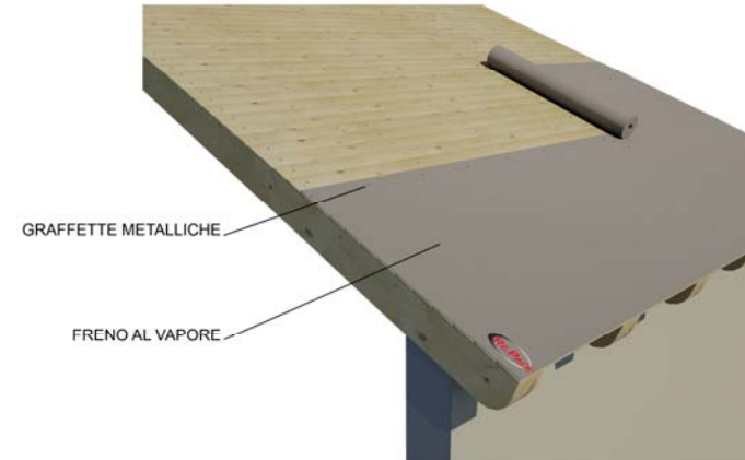
2) STESURA FRENO AL VAPORE
