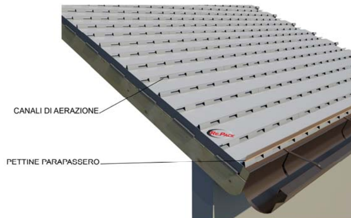
7) INSTALLAZIONE PETTINE PARAPASSERO
