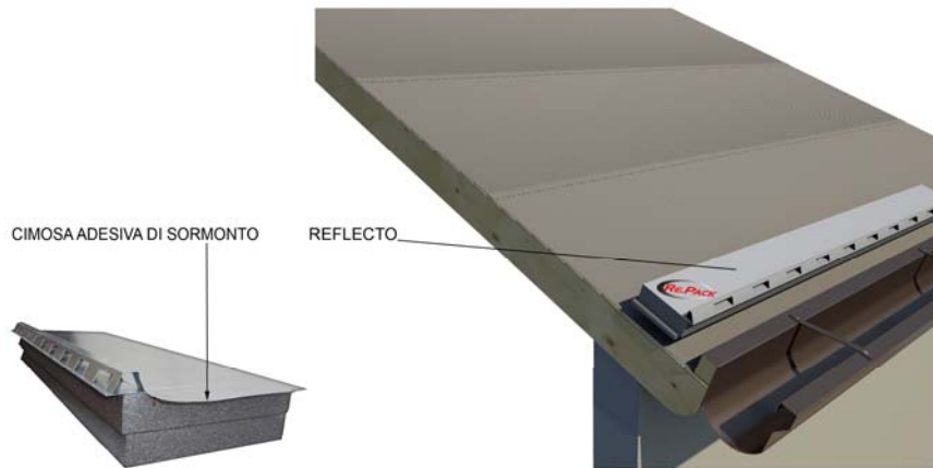
5) PANNELLO DI PARTENZA GRONDAIA
