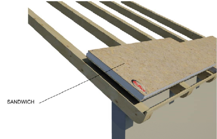
2) INSTALLAZIONE PANNELLO DI PARTENZA GRONDAIA
