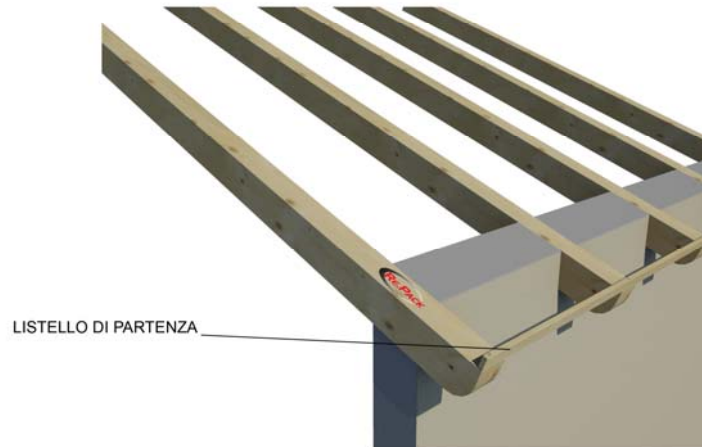
1) INSTALLAZIONE LISTELLO DI PARTENZA
