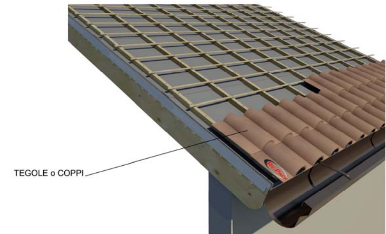
8) ANCORAGGIO TEGOLE o COPPI
