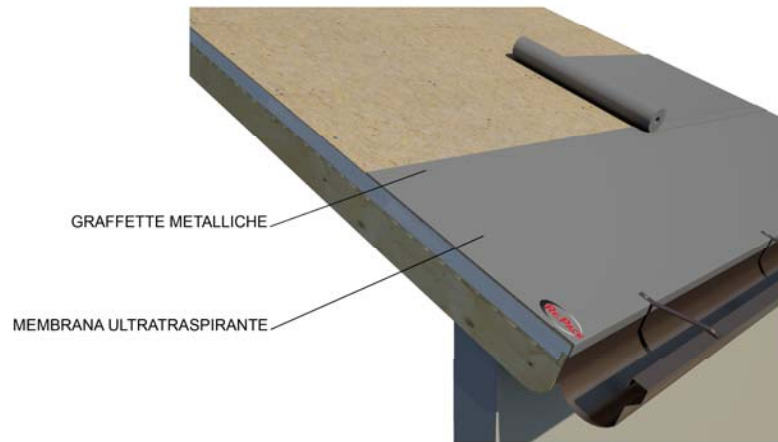
5) STESURA MEMBRANA ULTRATRASPIRANTE
