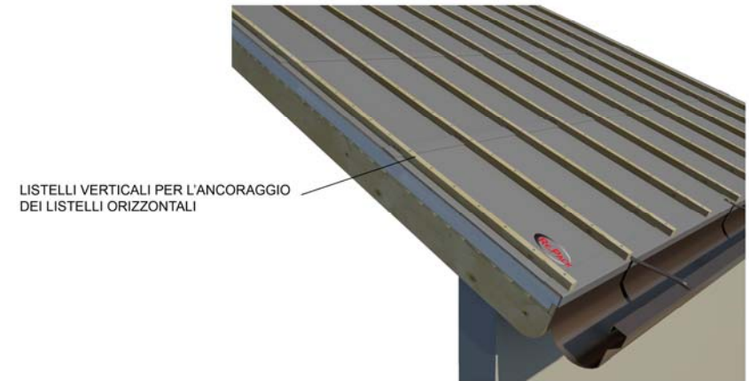
6) MONTAGGIO LISTELLI
