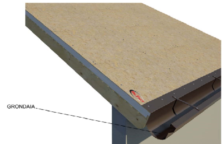
4) INSTALLAZIONE GRONDAIA
