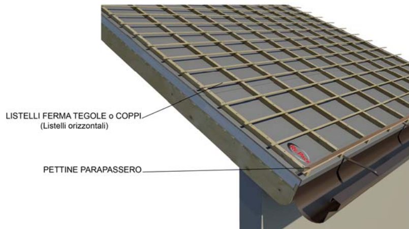
7) MONTAGGIO LISTELLI A PASSO TEGOLE o COPPI
